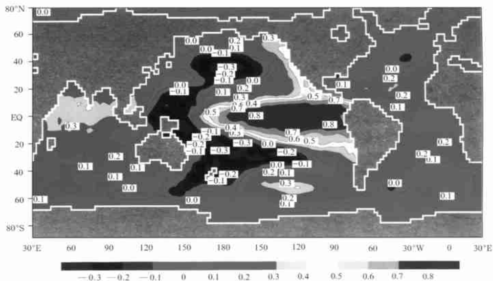
图 11 1871-1997 年逐月 Niño 3 区指数与全球 SST 距平的相关系数分布
