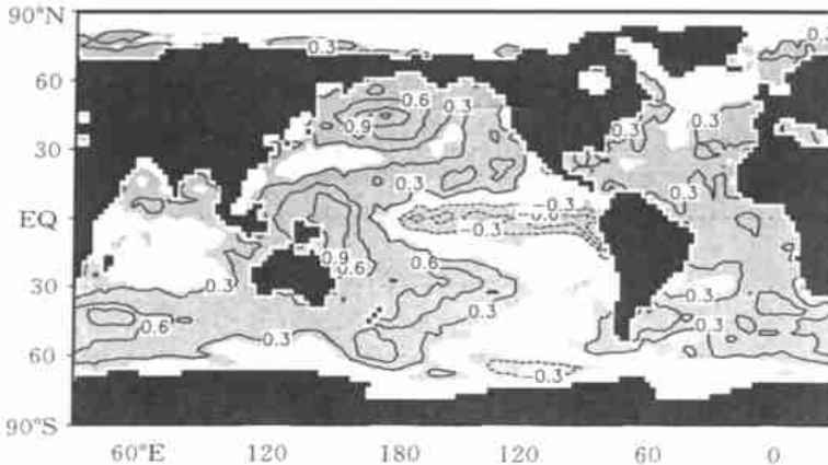
图 7 西太平洋暖池区极端冷、暖月份 SST 差值场的合成分析 (单位: ^{\circ}\text{C} ; 等值线间隔为 0.3; 阴影区表示温度变化幅度超过 \pm 0.2^{\circ}\text{C} )
