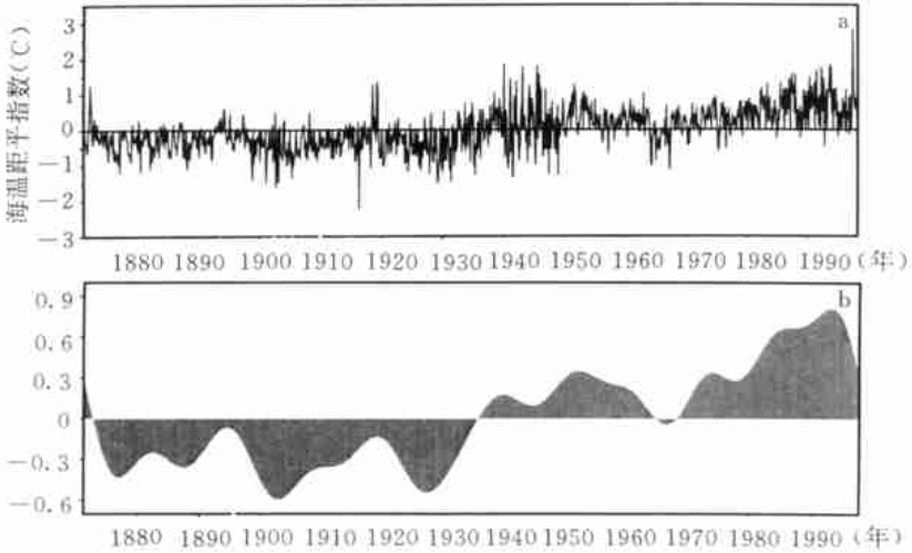
图 9 南印度洋(47.5~35.5 E, 42.5~77.5 S)区域平均月 SST 距平指数序列(a)及其滤掉 10 a 以下尺度变率后的结果(b) (单位: )
