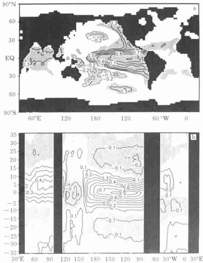
图 6 Niño 3 区指数序列与全球 SST 距平的相关分布型(a)及其与赤道 SST 距平的超前(落后)相关,纵坐标的负(正)值表示其它大洋超前(落后)于 Niño 3 区指数(b);(阴影区表示信度超过 95%)
