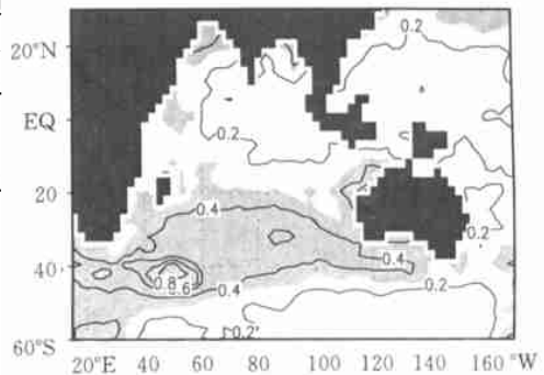
图 1 印度洋年平均海温标准差分布 (单位: ^{\circ}C , 阴影区表示标准差大于 0.4)
