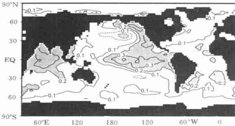
图 4 标准化后的赤道印度洋 SST 距平指数与全球 SST 的回归系数分布 (阴影区表示回归系数大于 0.2; 单位: \delta R )
