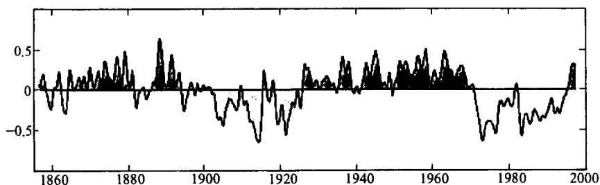
图3 北大西洋北部 (45~65°N, 20~60°W) 区域平均 SST 距平时间序列 (引自文献[10])
