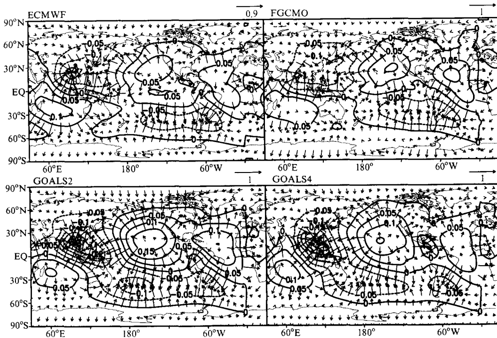
图4 同图3, 但为7月份的情况
