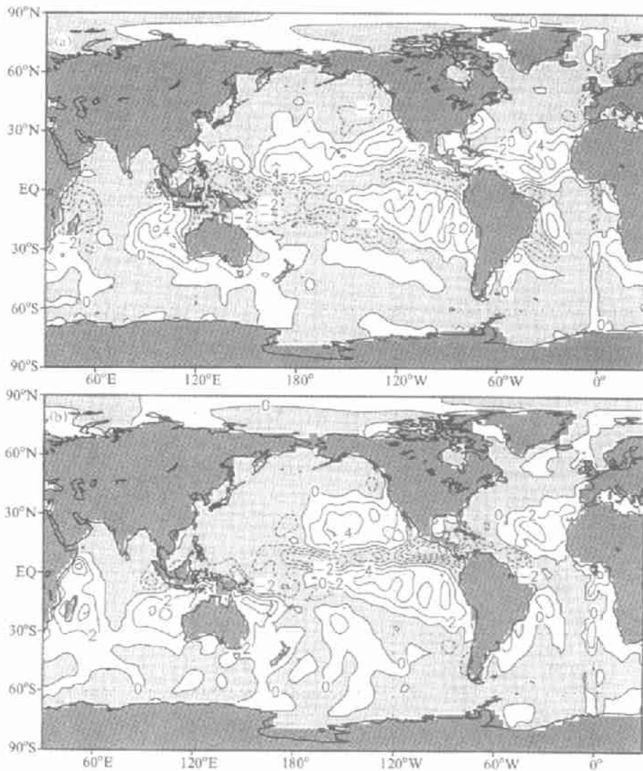
图8 利用实测 SST 强迫 CCM3 得到的水通量分布 (单位: \text{mm d}^{-1} ) (a) 1月; (b) 7月
