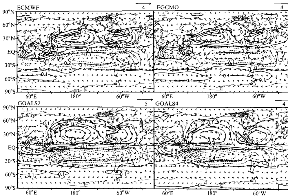
图2 同图1, 但为7月份的情况
