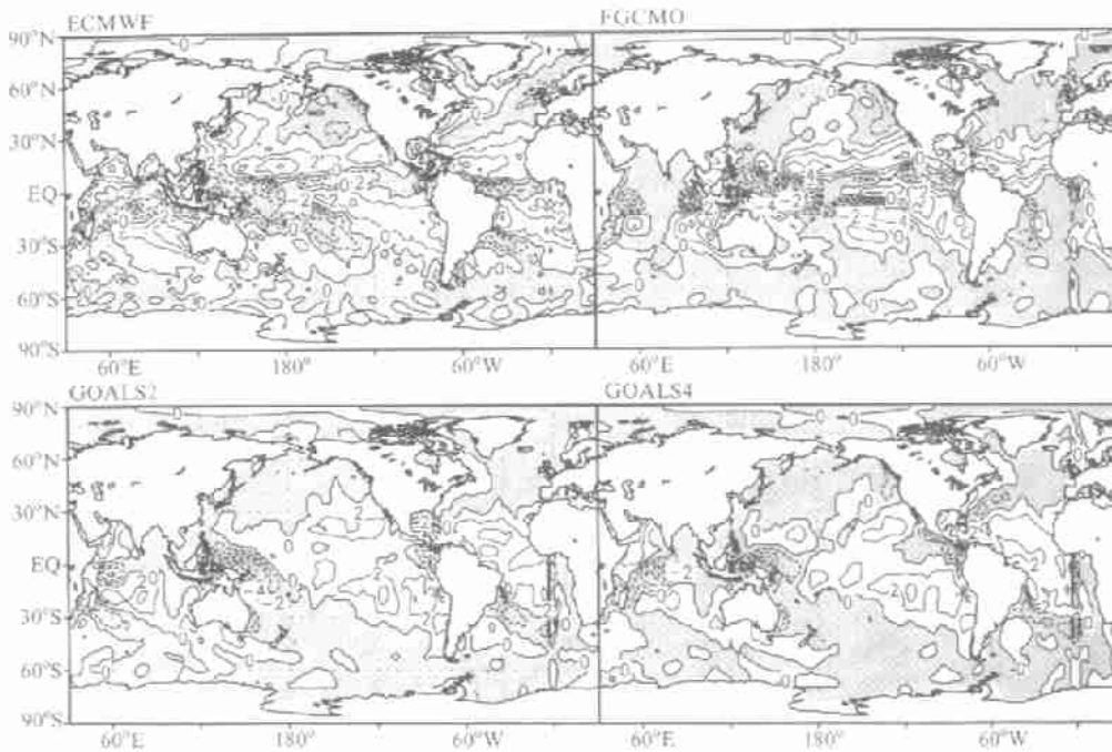
图 5 根据 ECMWF 资料估算和耦合模式模拟的 1 月份全球海气间水通量交换 (单位: \text{mm d}^{-1} )
