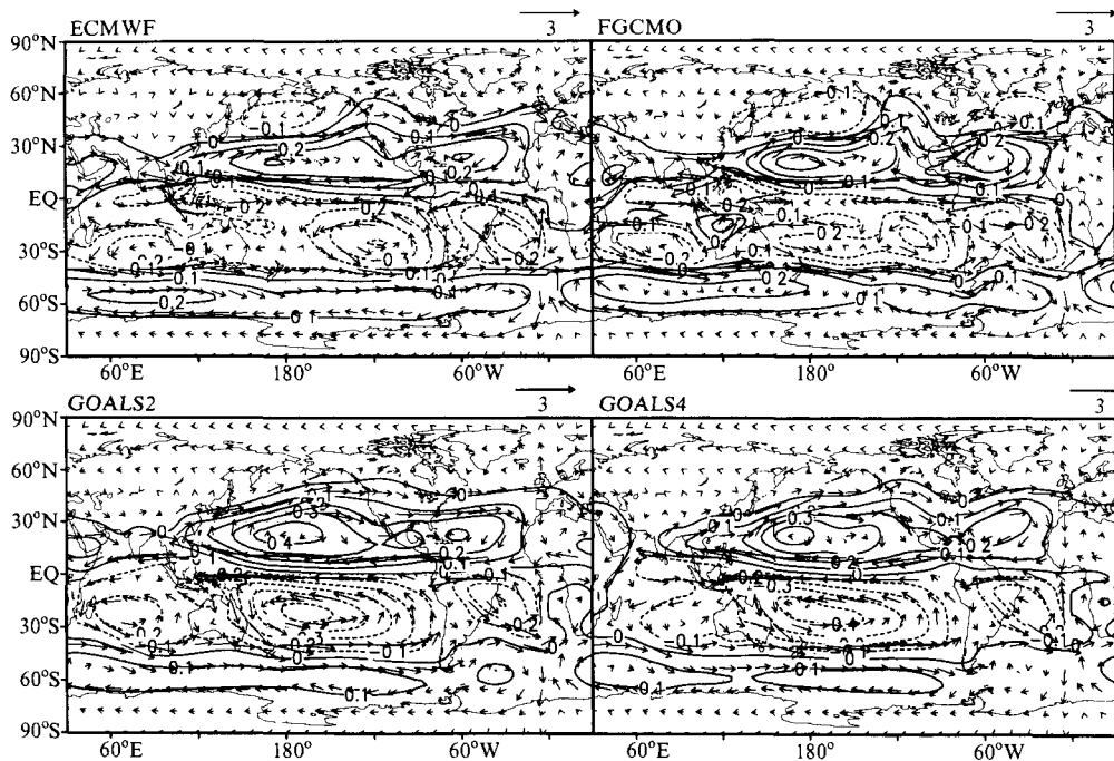
图1 1月份垂直积分的水汽通量场的流函数(细等值线, 单位: 10^6 \text{ m}^3 \text{ s}^{-1} , 等值线间隔为0.1)和无辐散的水汽通量场(矢量, 单位: 10^2 \text{ kg m}^{-1} \text{ s}^{-1} )
