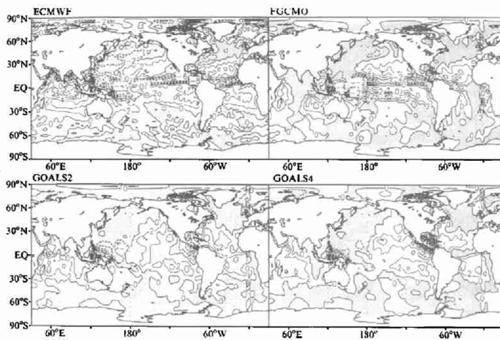
图6 同图5, 但为7月份的结果
