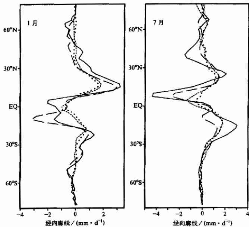
图7 1月份和7月份纬向平均的全球海气间水通量交换的经向廓线 实线: ECMWF; 长虚线: FGCM-0; 短虚线: GOALS-2; 点线: GOALS-4
